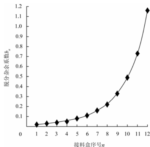
图 4 脱分杂余系数 b_n 曲线拟合
