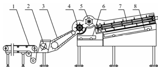
1. 输送带 2. 喂入搅搅 3. 输送槽 4. 切流滚筒 5. 辅助喂入轮 6. 切流分离接料盒 7. 纵轴流滚筒 8. 纵轴流分离接料盒
