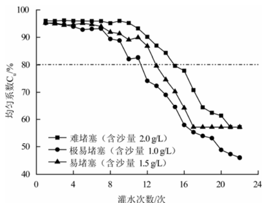
b. 灌水器均匀系数变化
