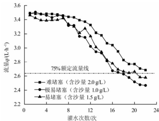
a. 灌水器流量变化
