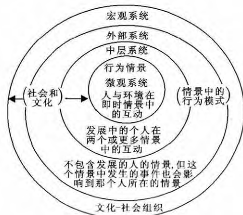
图 1 生态系统图
