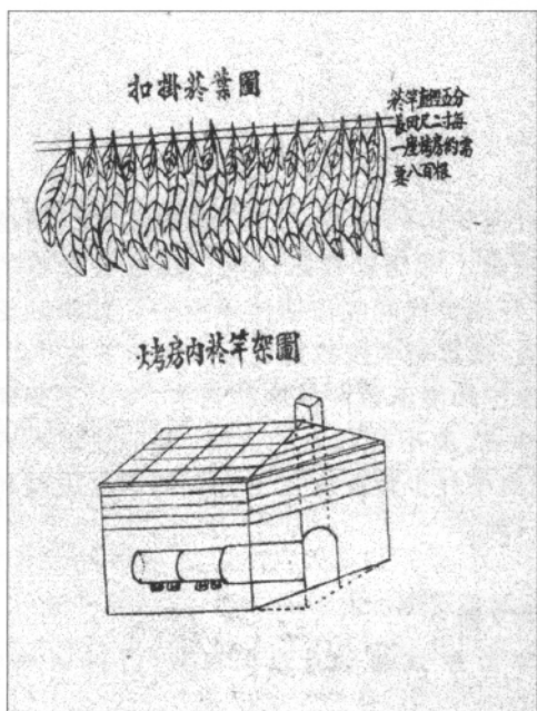
扣挂烟叶及烤房内烟杆架图
