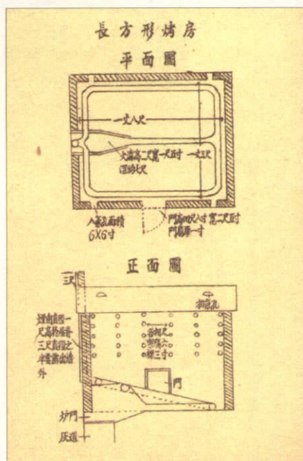
长方形烤房示意图
